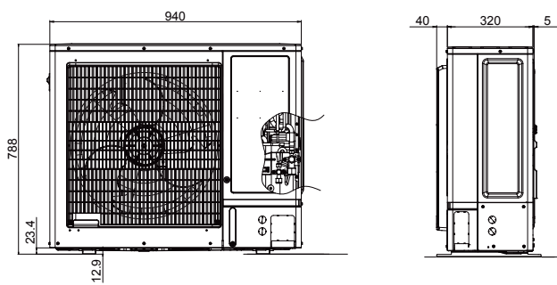
Vista frontale
