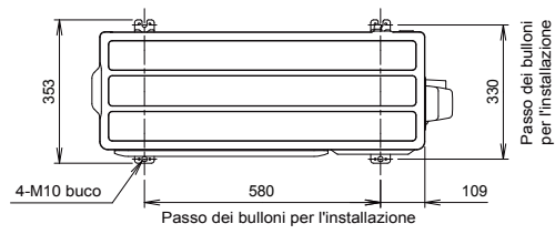
Vista dall'alto
