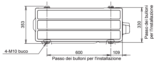
Vista dall'alto
