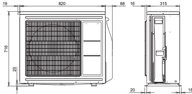
Vista frontale
