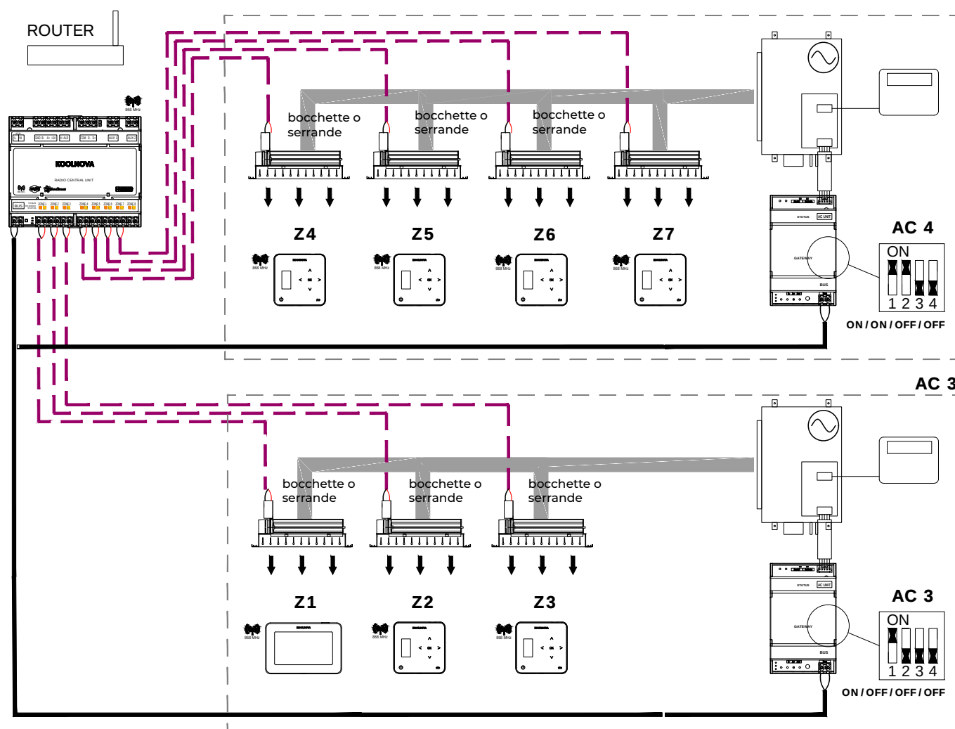
Schema collegamento elettrico e di principio
